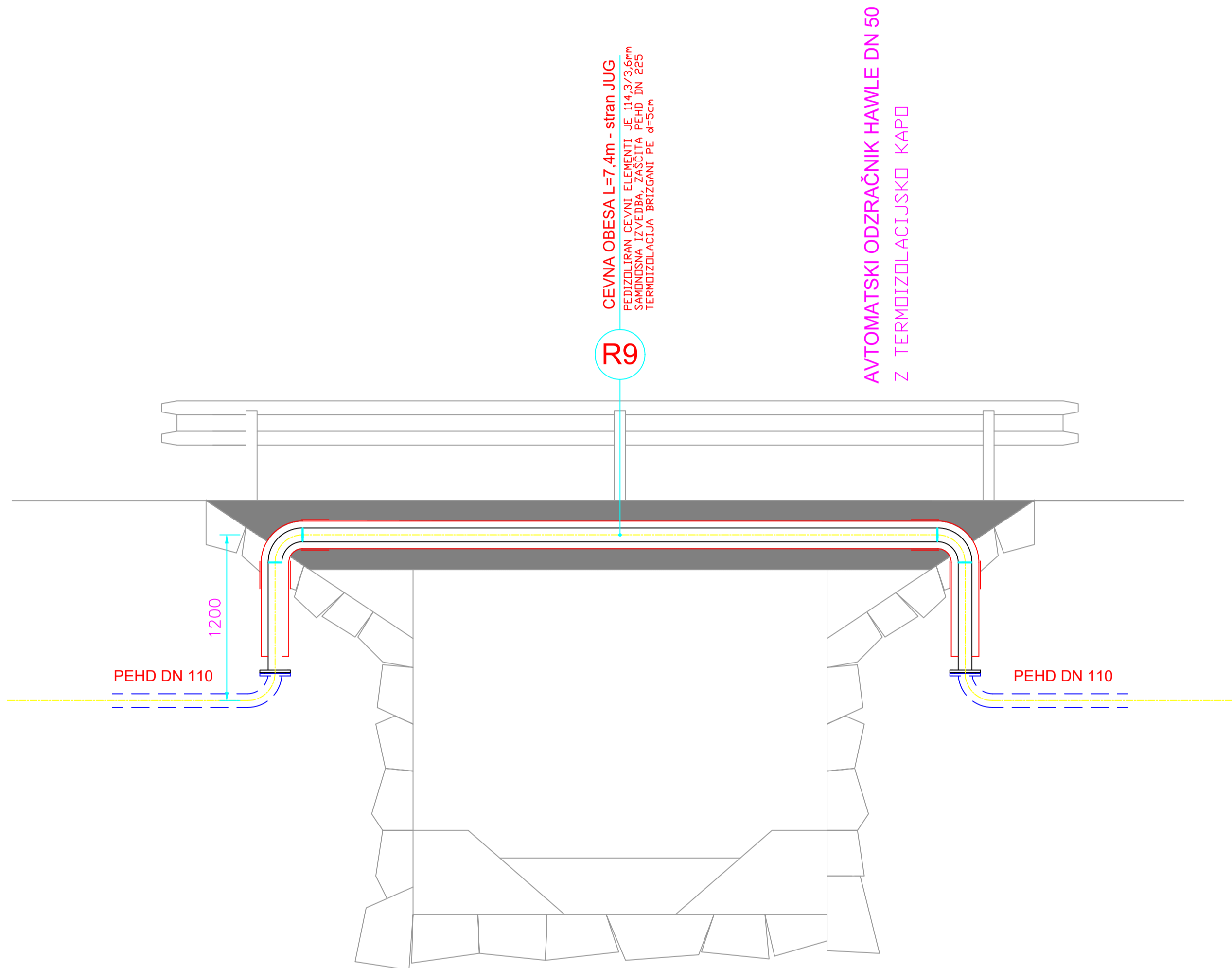
PREREZ A-A
