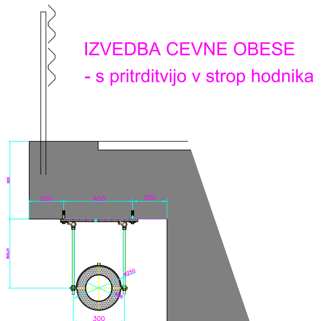
PREREZ A-A
